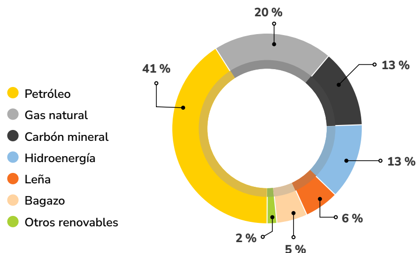
Figura 4.1 | Matriz energética de Colombia, 2021
