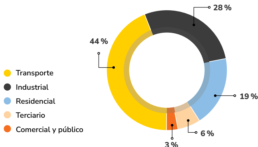
Figura 4.2 | Consumo energético de Colombia por sector, 2020
